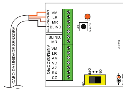
UNIDADE TRANSMISSORA
