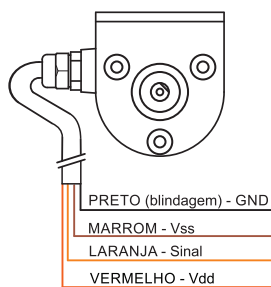
UNIDADE SENSORA
