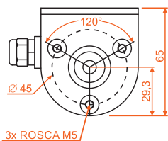
UNIDADE SENSORA
